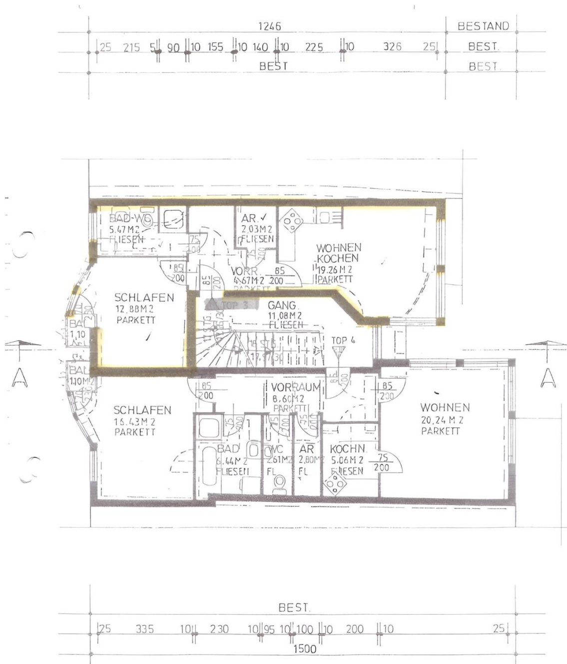
Grundriss
