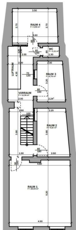
OBERGESCHOSS
