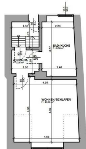
DACHGESCHOSS
