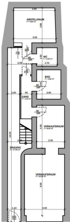
ERDGESCHOSS
