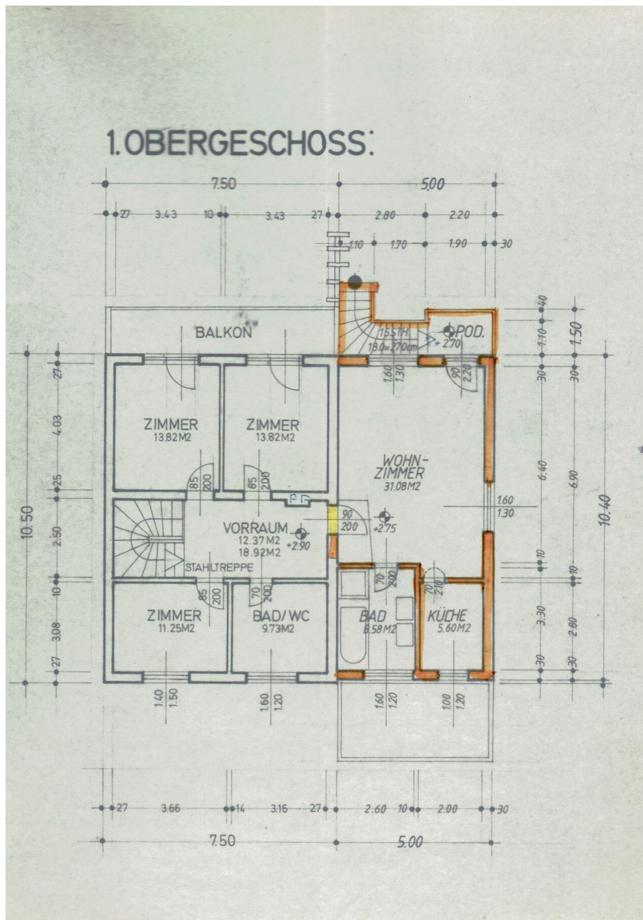
Obergeschoss
