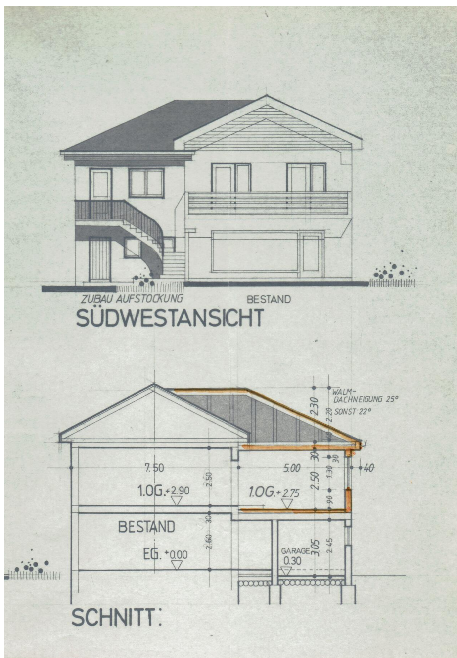
Südwestansicht
