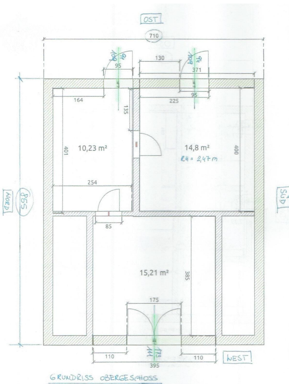
Grundriss Obergeschoss
