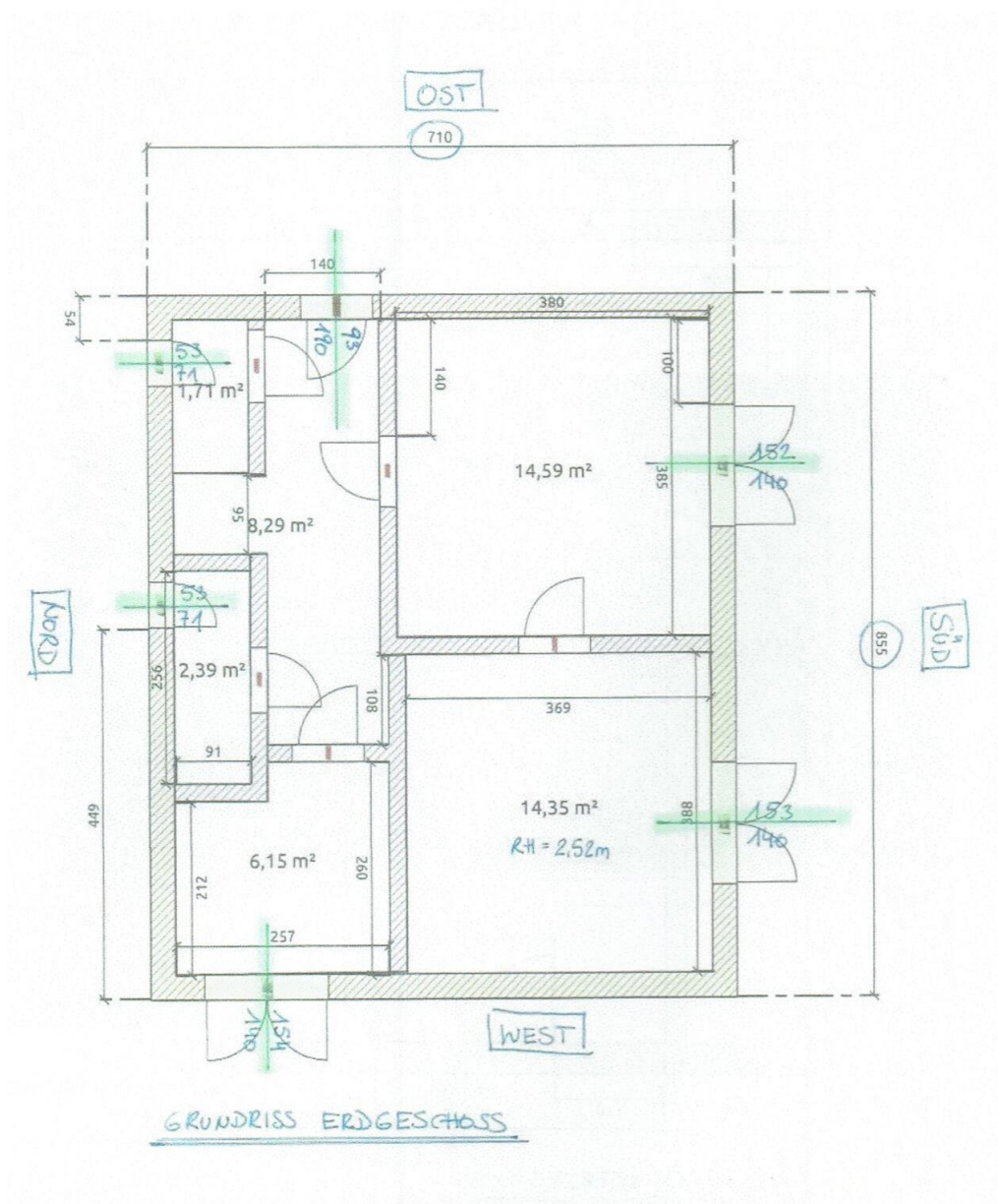
Grundriss Erdgeschoss
