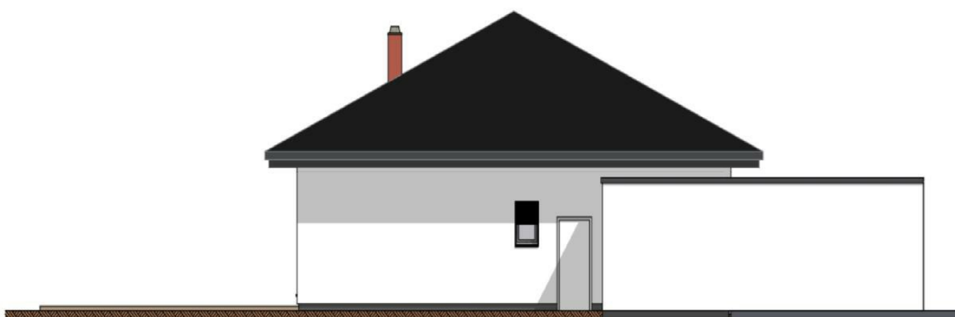
ANSICHT MASSTAB 1:100 OSTEN
