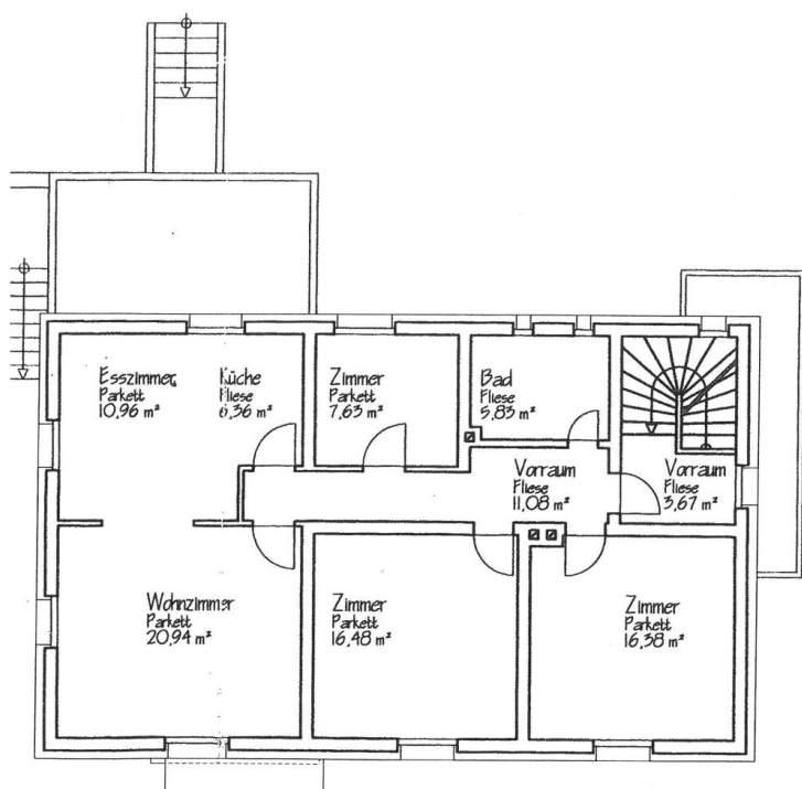
2. OBERGESCHOSS BESTAND
