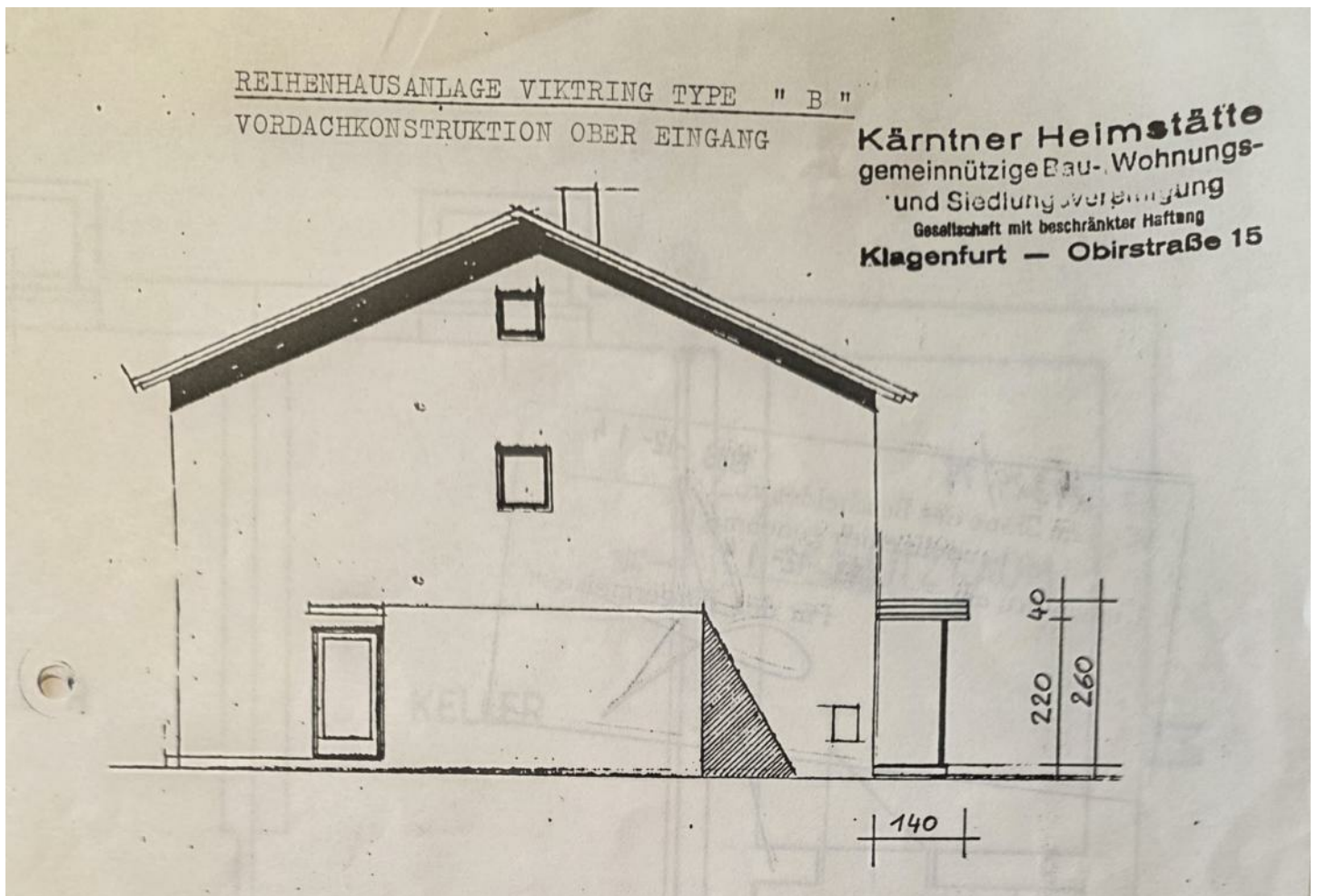
Südansicht
