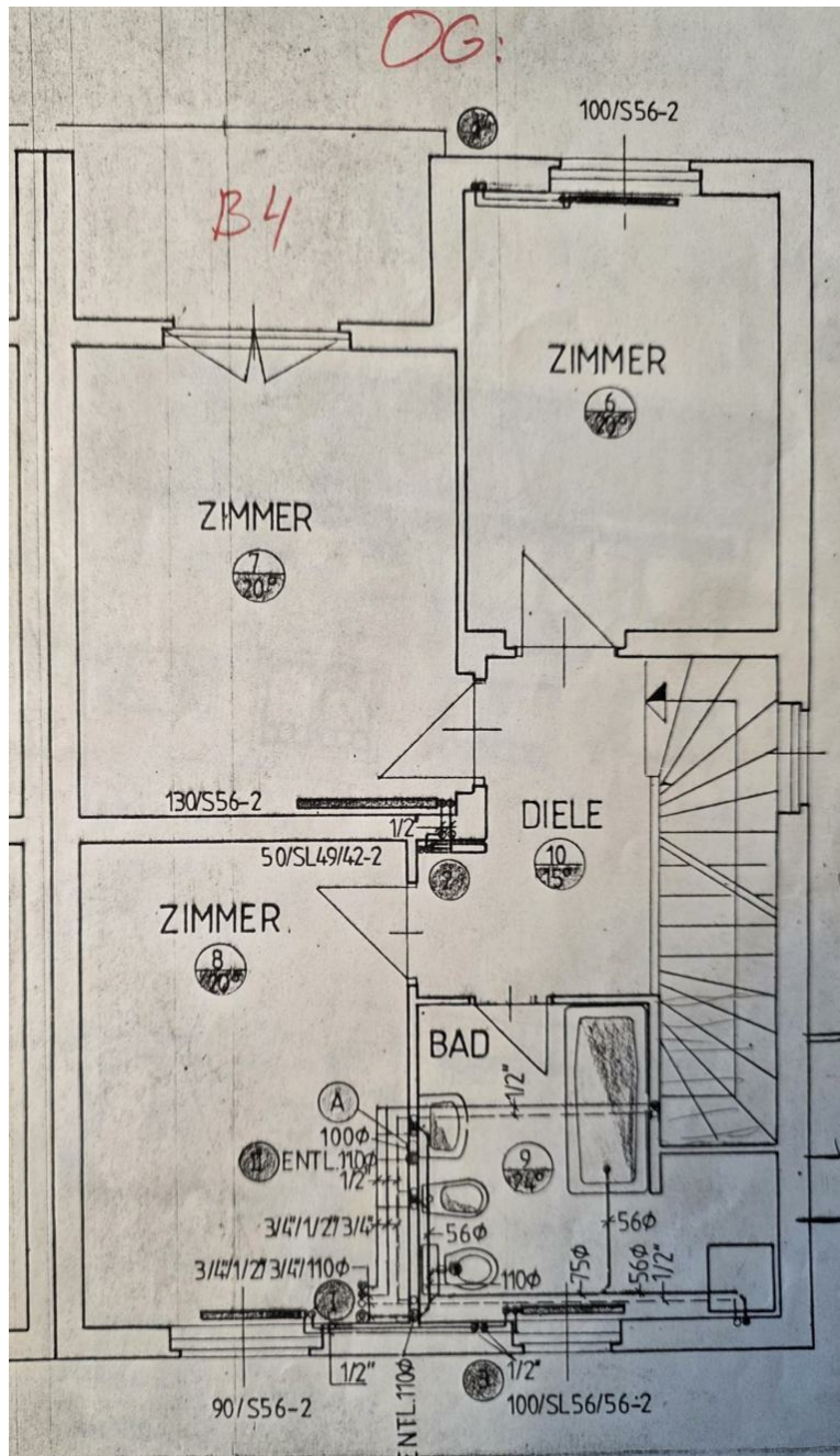
Obergeschoss
