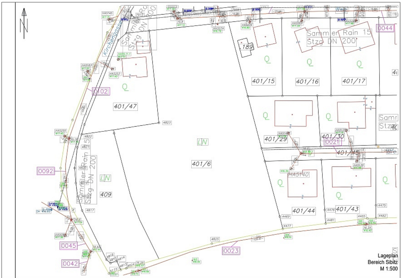
Kanal und Wasserleitungsplan
